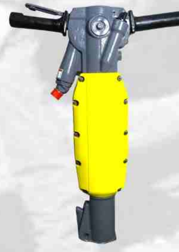
TEX 230 PE
